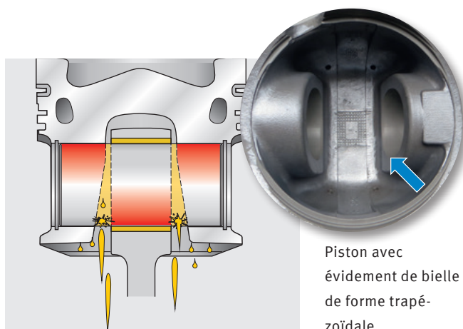
Piston avec évidement de bielle parallèle
